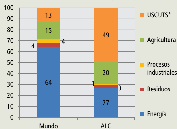
Gráfico 5.5 Mundo y América Latina y el Caribe. Emisiones de Gases de Efecto Invernadero (GEI) por sector.
